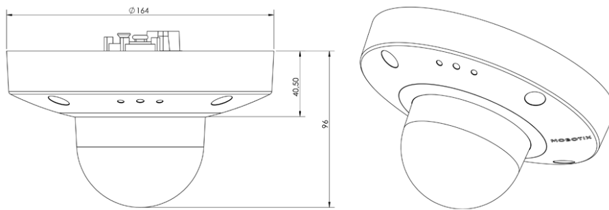
Fig. 1: D71: Todas las medidas en mm
